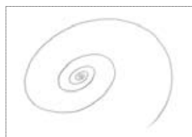
図13 渦巻きの線
